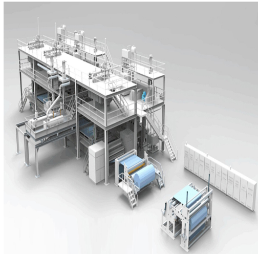
Type: SSMMS Speed: 600m/min Fibre Denier:1.6-1.8D
