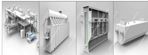
Type: SSMMS Speed: 600m/min Fibre Denier:1.6-1.8D
