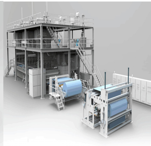
Type: SSS Speed: 600m/min Fibre Denier:1.6-1.8D
