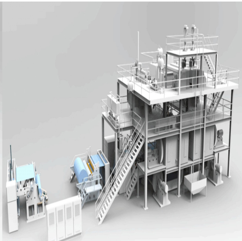
Type: SS Speed: 350m/min Fibre Denier:1.6-1.8D
